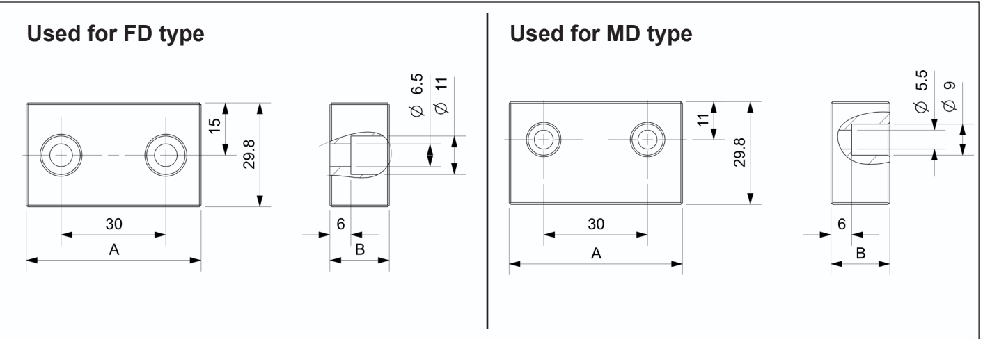
50RZ-B 型软爪 | 50RZ-B type soft jaw
