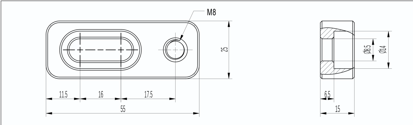
88DW 工件定位器 | 88DW work positioner
