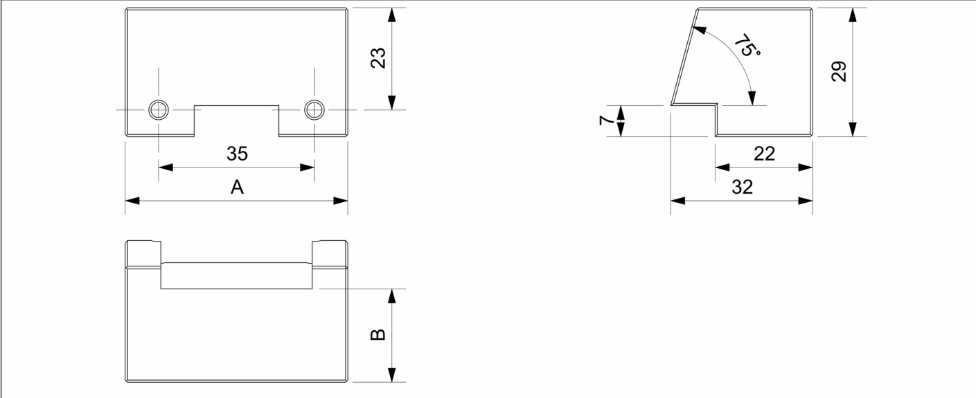
50RZ-C 型软爪 | 50RZ-C type soft jaw
