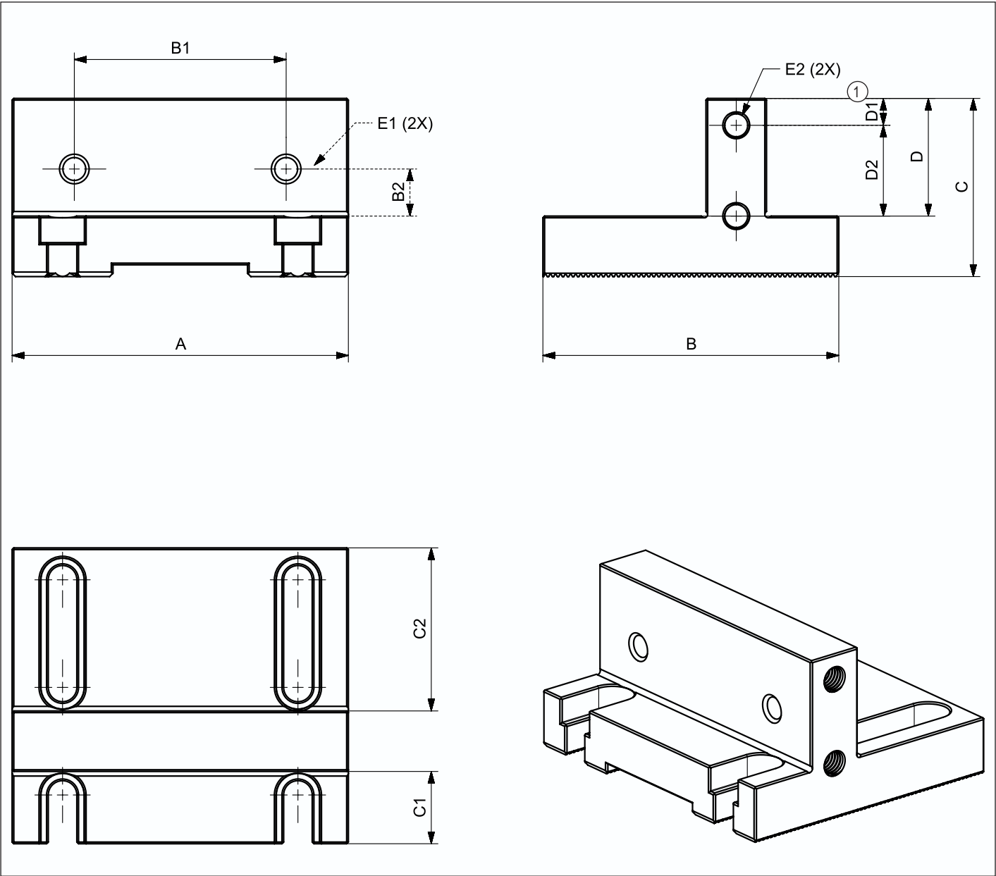
① 用于固定挡块
