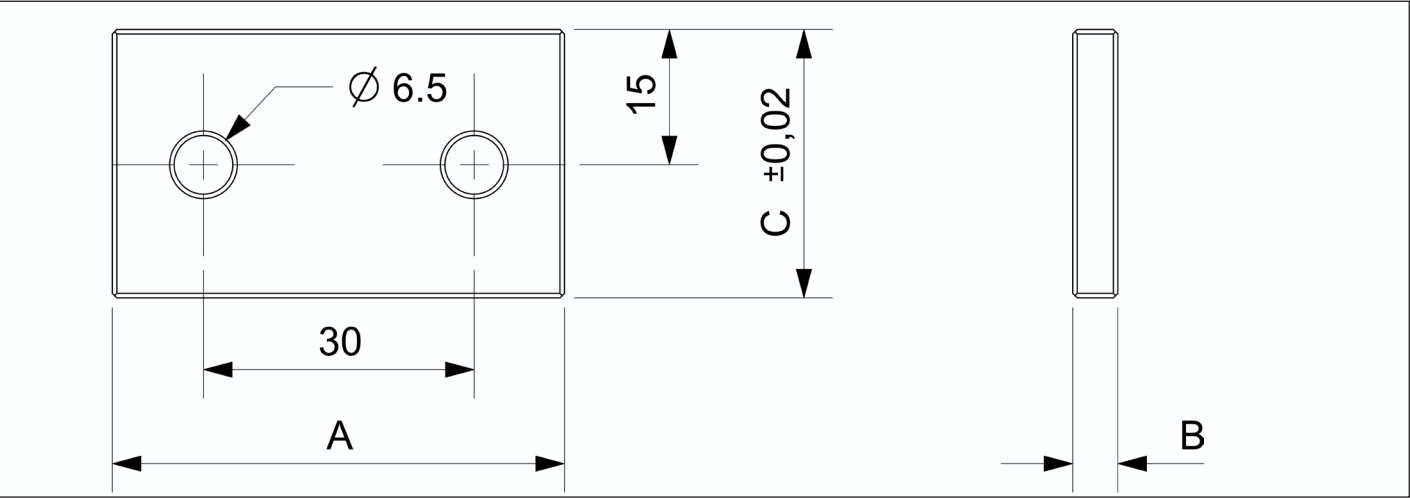
50DP 平行垫块 | 50DP Parallel gasket
