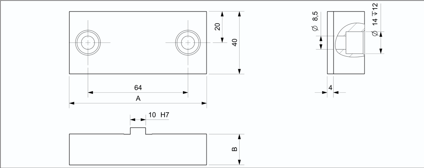
88RZ-A 型软爪 | 88RZ-A type soft jaw
