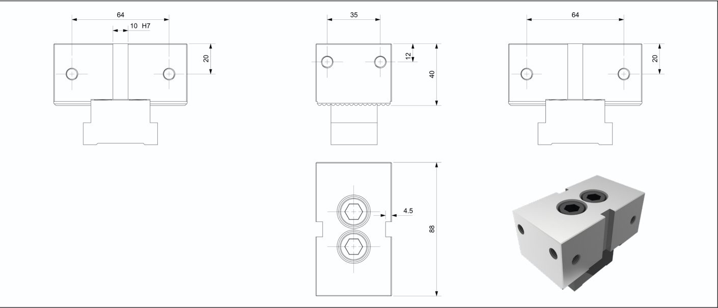
88G 固定钳口 | 88G type unidirectional clamping jaw
