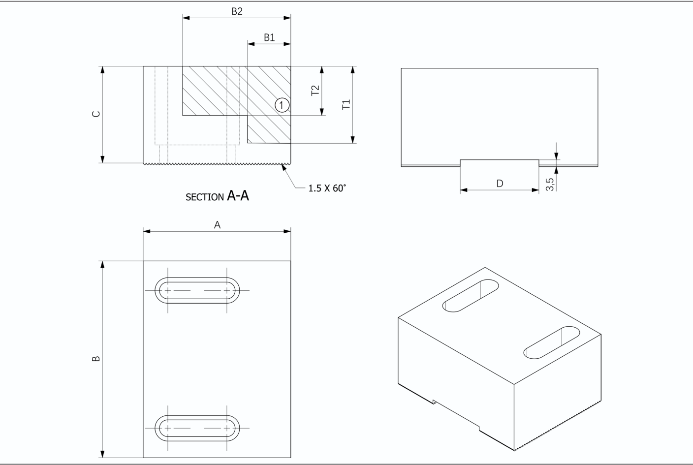
① 工作区域 ① Work surface
