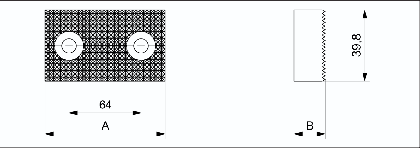
88C 齿型钳口 | 88C serrated Jaw
