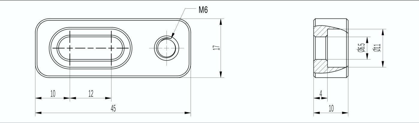
50DW 工件定位器 | 50DW work positioner
