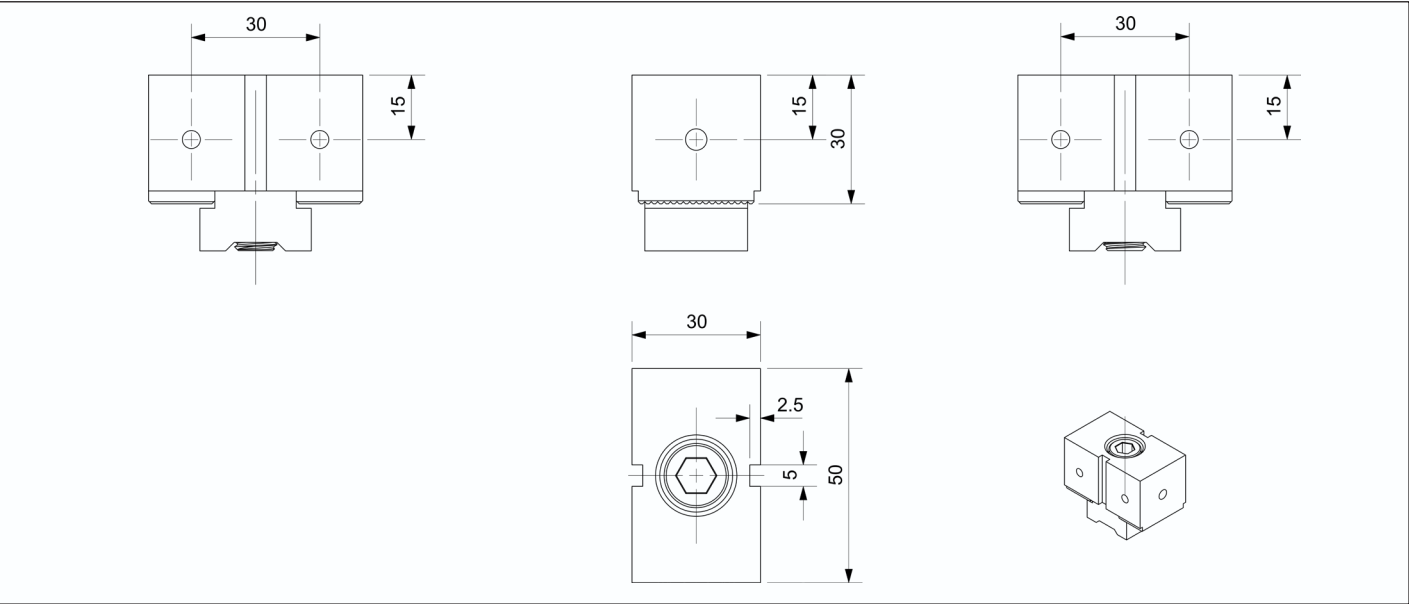
50SG 固定钳口 | 50SG type fixed clamping jaw
