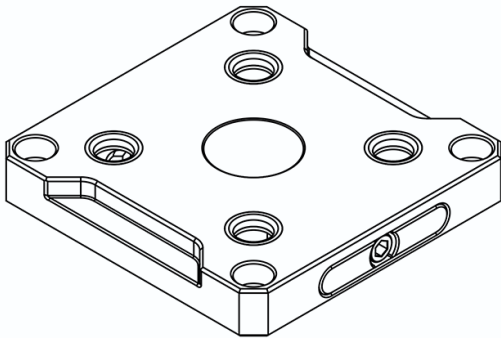
① 96 型拉钉锁紧接口 Type 96 positioning interface
