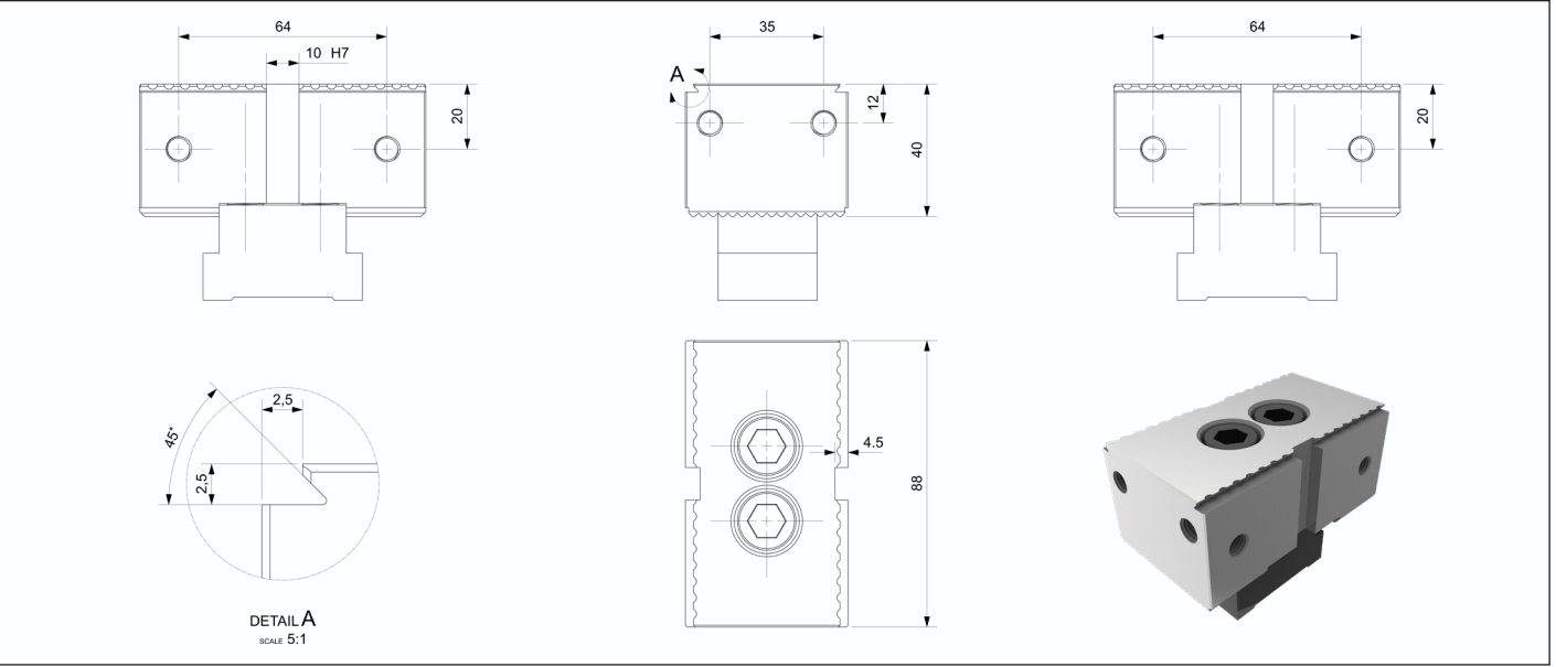
88G-T 锯齿型固定钳口 | 88G-T Jagged fixed jaw
